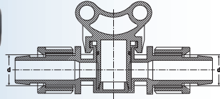
MİNİ VANA Damlama Mini Valve Dripline
