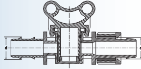
MİNİ VANA Kurtağzı - Damlama Mini Valve Barbed - Dripline
