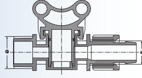
MİNİ VANA Erkek - Damlama Mini Valve Male - Dripline
