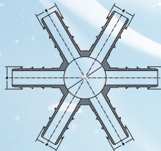
KURTAĞZI ÇOKLU DAĞITIM NİPELİ Barbed Multicoupling
