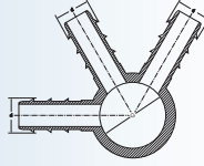
KURTAĞZI ÇOKLU DAĞITIM NİPELİ Barbed Multicoupling
