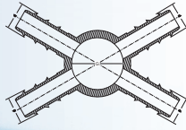
KURTAĞZI ÇOKLU DAĞITIM NİPELİ Barbed Multicoupling
