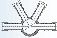
KURTAĞZI ÇOKLU DAĞITIM NİPELİ Barbed Multicoupling
